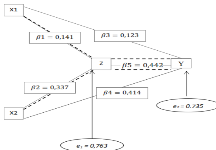
Gambar 2. Model Analisis Jalur
