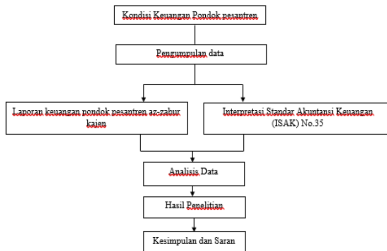
Gambar 1. Kerangka Berfikir
